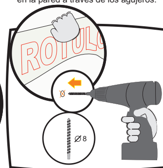
5.- Retirar la plantilla de la pared y realizar un agujero en cada marca de las varillas.
