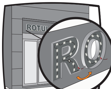
7.- Una vez colocadas todas, conectar cada letra con la siguiente a través del cable lateral.
