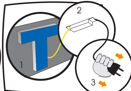
8.- Colocar los frontales de metacrilato y conectar la última letra al transformador led y éste a la corriente 220V.
