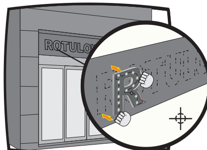
6.- Pegar o atornillar todas las letras haciendo coincidir las esquinas de las letras con las marcas de la pared.
